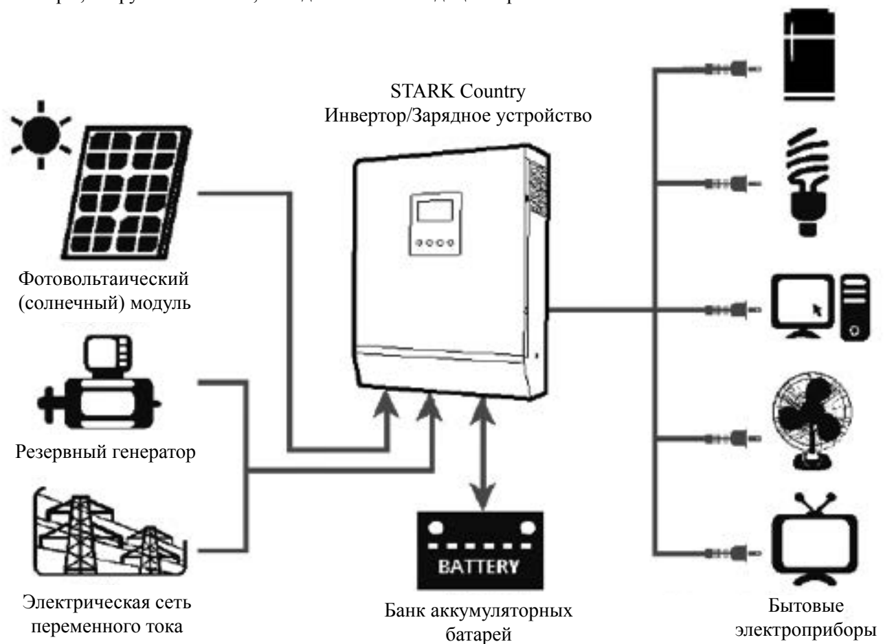
Рис. 1 Схема системы электропитания
